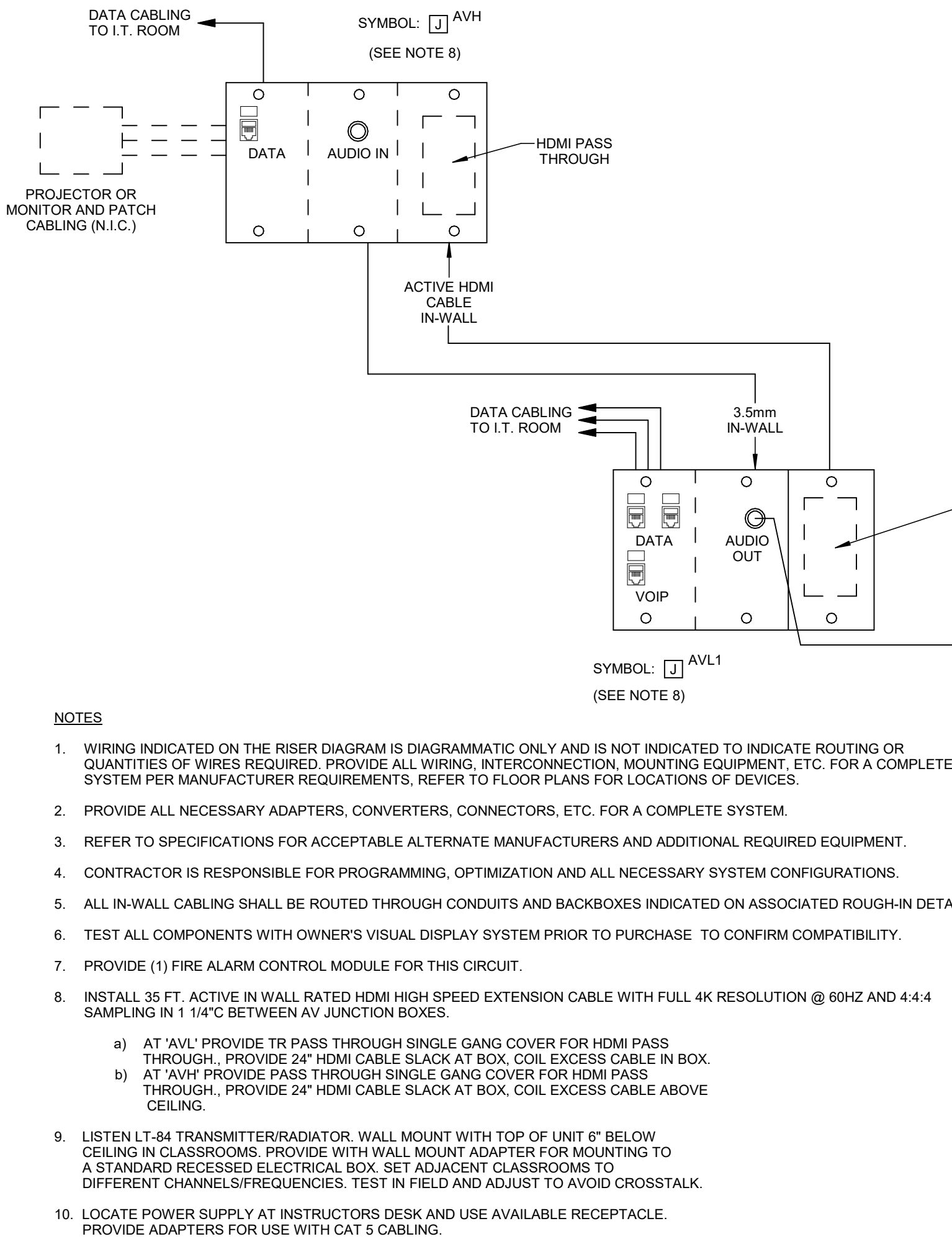
2 TYPICAL INTERACTIVE PROJECTOR AV WIRING DETAIL N.T.S.
